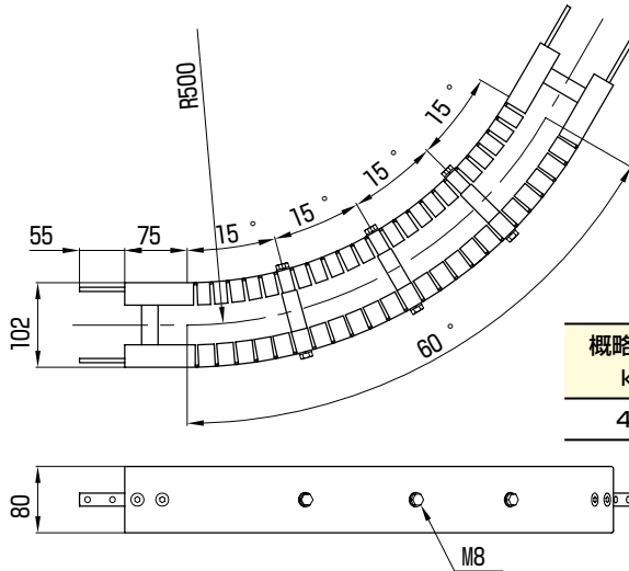
■ 60° (コード:36UTNCFN060)
