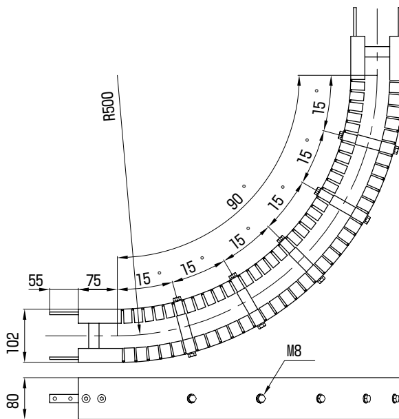
■ 90° (コード:36UTNCFN090)
