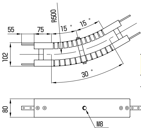
■ 30° (コード:36UTNCFN030)
