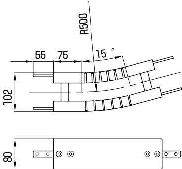
■ 15° (コード:36UTNCFN015)
