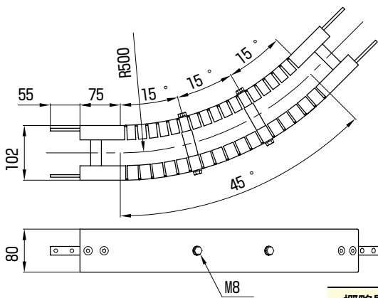
■ 45° (コード:36UTNCFN045)
