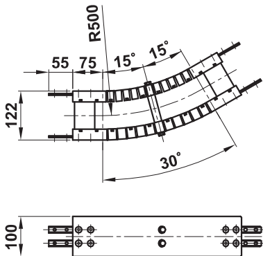
カーブフレームユニット(60度) Curve Frame Unit ( 60-degree )
