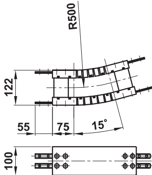
カーブフレームユニット(30度) Curve Frame Unit ( 30-degree )
